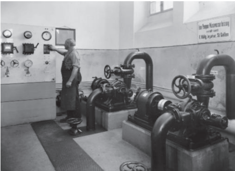
Abb. 30: Die Pumpen der neuen Heizung (Bild: Marthaler, Stella-Photo, Einsiedeln).
